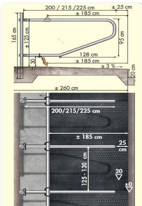
Varianta 1: Dimensiuni de asamblare pentru cuseta universală instalată pe un cadru de suport, pentru animale grele, pe un singur rand
