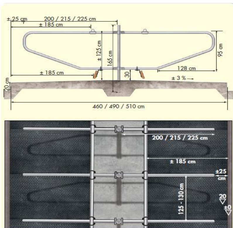
Varianta 1: Dimensiuni de asamblare pentru cuseta universală instalată pe cadru de suport, pe două randuri, pentru animale grele (dimensiunile sunt neobligatorii).
