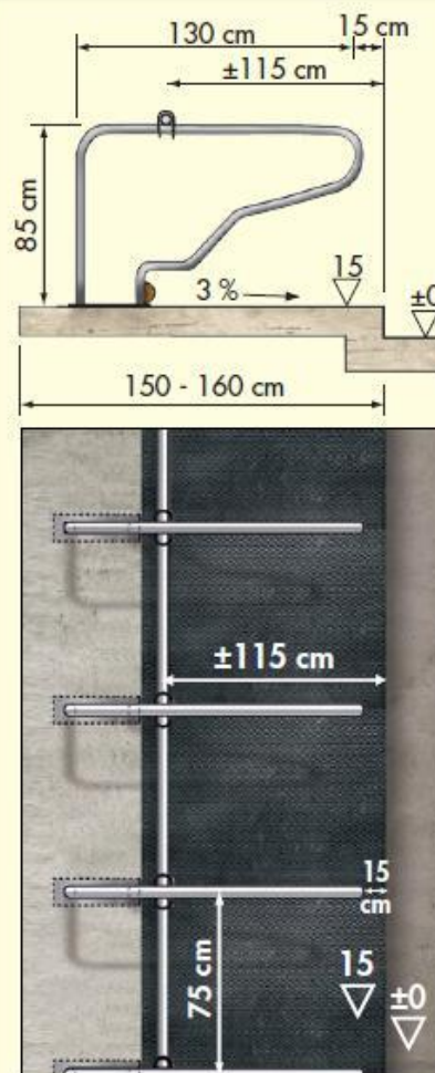
Dimensiunile de instalare a sistemului Clasic pentru vitei (dimensiunile sunt orientari neobligatorii)
