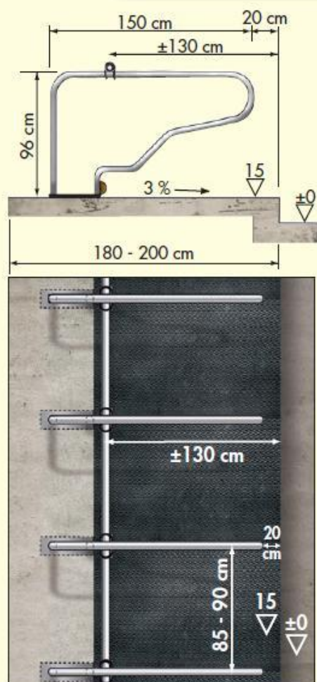
Dimensiunile de instalare a sistemului Clasic pentru vaci tinere (dimensiunile sunt orientari neobligatorii)
